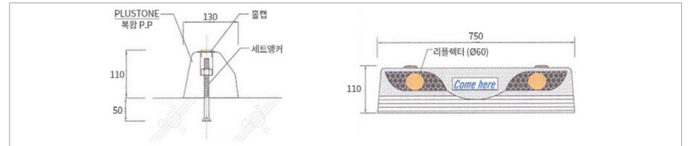
카키퍼 단면상세도
