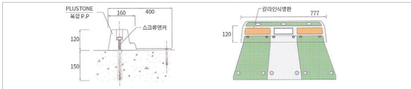
외부용카스토퍼 단면상세도
