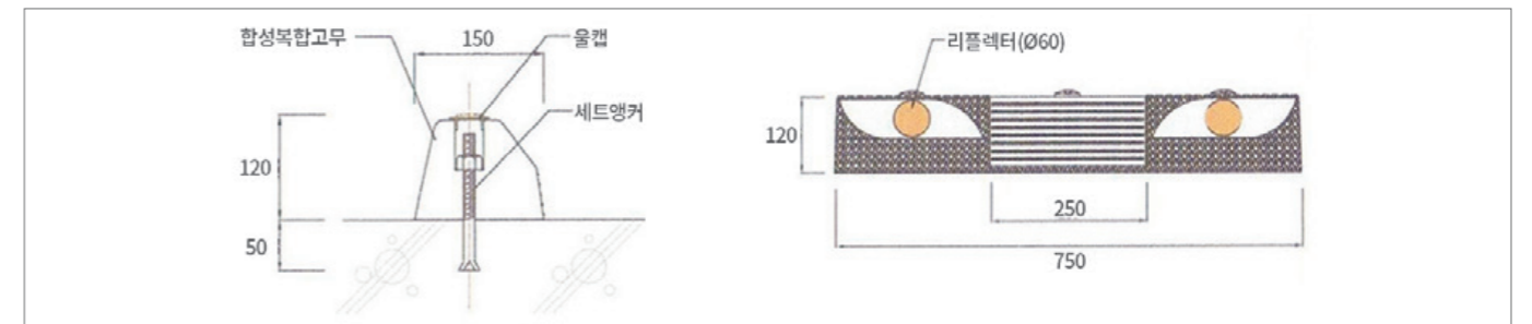
고무카스토퍼 단면상세도
