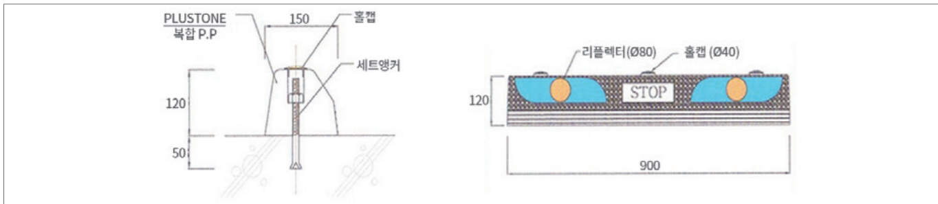
파킹가드 단면상세도
